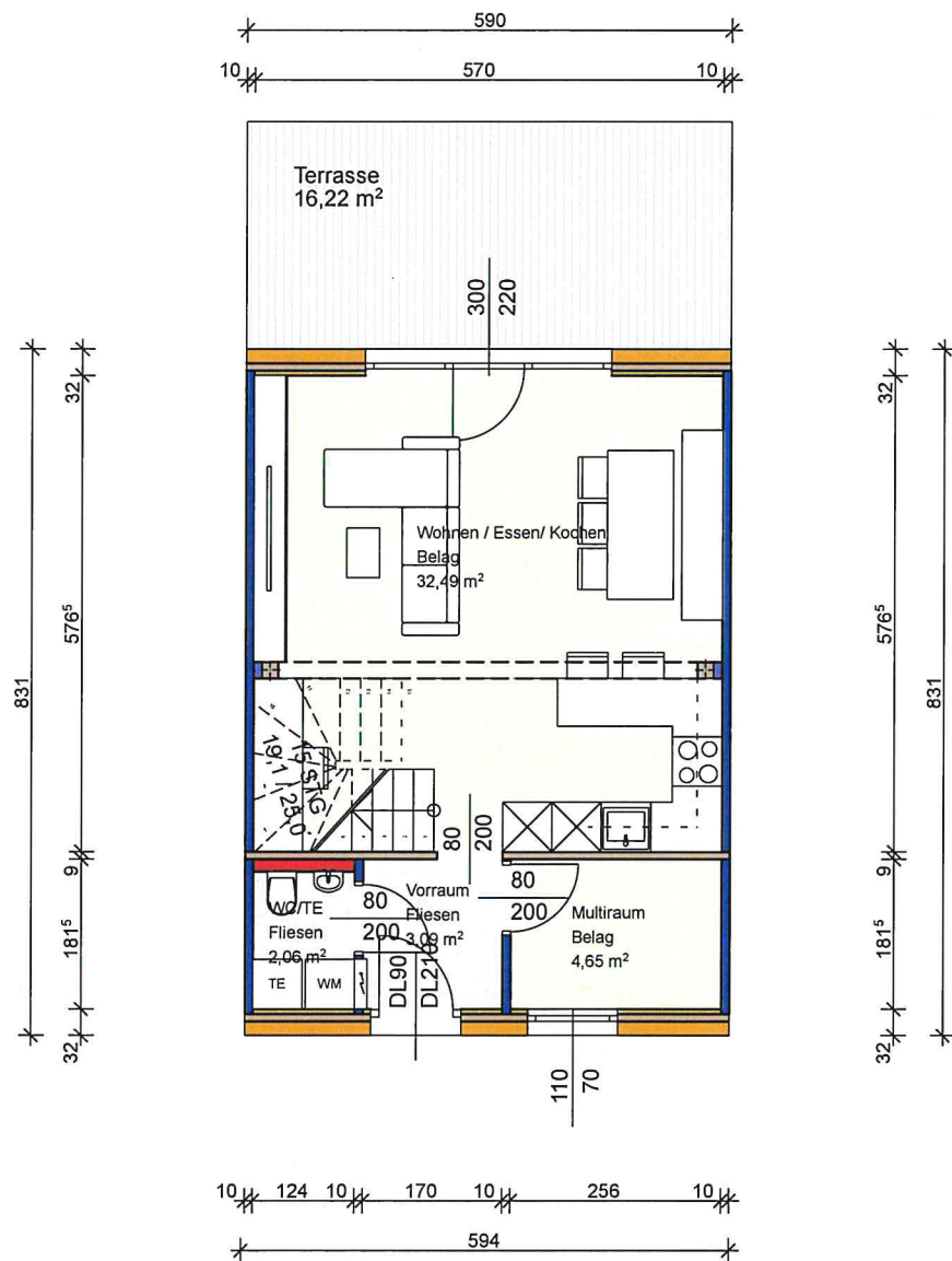
TYP 88 ERDGESCHOSS M1:100
